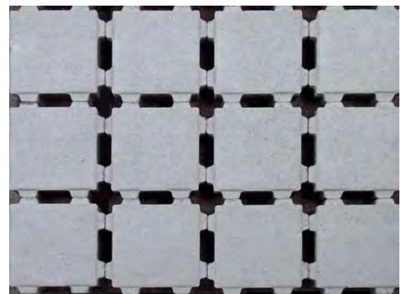
Ökopflaster 20x20 cm, grau, Kreuzfuge, 3 cm Fugenbreite
