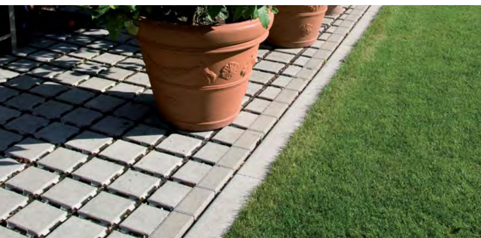
Ökopflaster 20x20 cm, grau, Drainfuge
