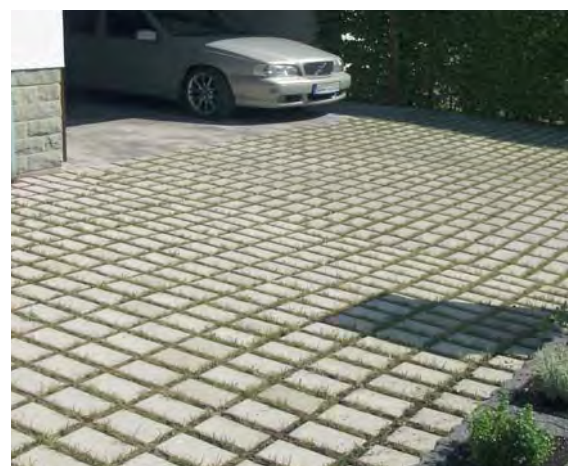
Ökopflaster 24x16 cm, grau, Rasenfuge
